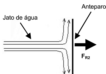
Fig.1b – Anteparo Plano
