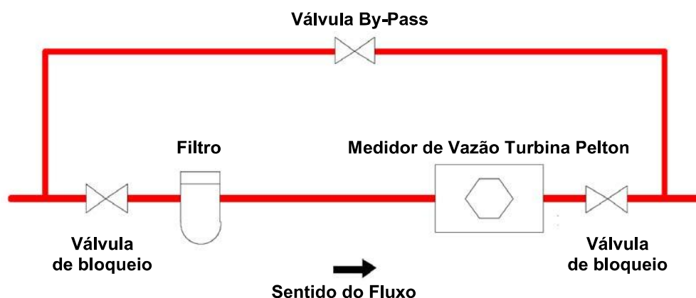
Fig. 4 – Esquema de Montagem
